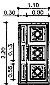
WOODEN DOOR SC=1:50 TYPE-3
