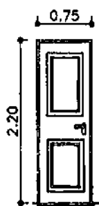
WOODEN DOOR SC=1:50 TYPE-2
