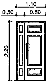
METAL DOOR SC=1:50 TYPE-1
