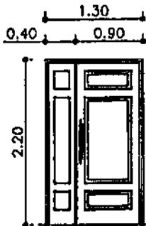
METAL DOOR SC=1:50 TYPE-2
